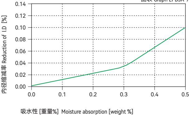
图表 Graph EPB5A-9
