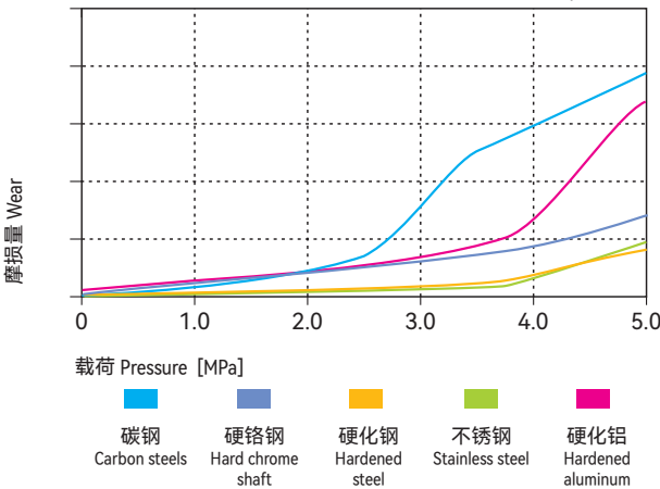
图表 Graph EPB25-8
