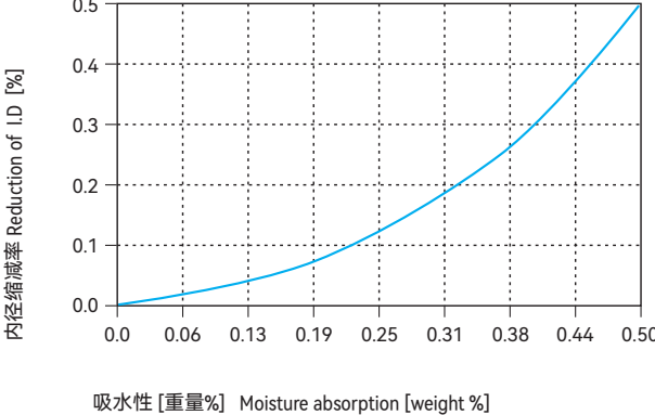
图表 Graph EPB1-9
